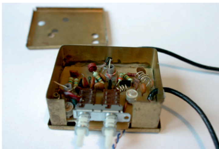
Przystawka do radia umożliwiająca podsłuch SB przystosowana do instalacji samochodowej
